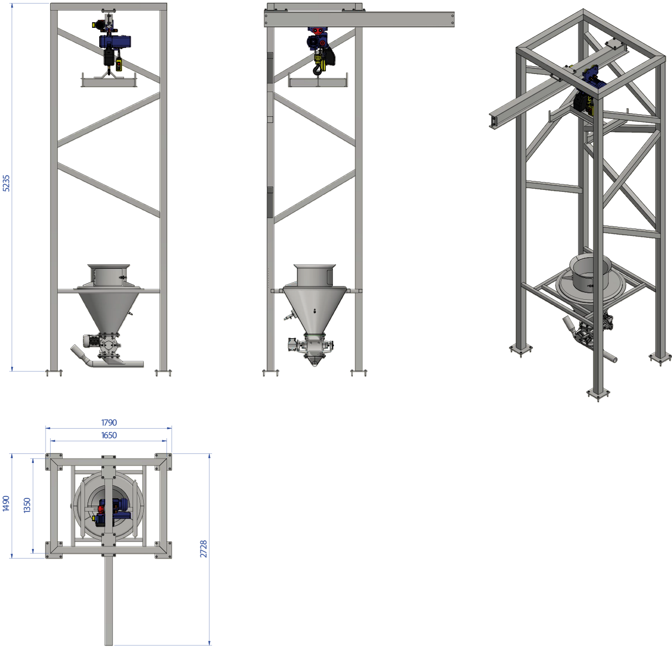
Dimensiones equipo Big bag con fondo fijo básico
