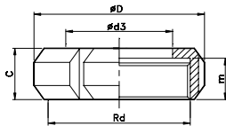
TUERCA SMS NUT SMS ECROU SMS
