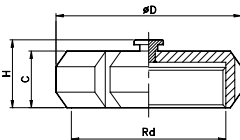
TUERCA CIEGA CON PIVOTE BLIND NUT WITH BOSS ECROU BOUC. AVEC PIVOT
