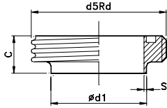
MACHO SOLDAR SMS WELDING MALE SMS NEZ À SOUDER SMS
