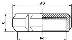
TUERCA CIEGA SMS BLIND NUT SMS ECROU BOUCHON SMS
