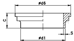
CASQUILLO SOLDAR SMS WELDING LINER SMS DOUILLE À SOUDER SMS
