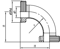
CODO 90° M/M SMS BEND 90° M/M SMS COUDE 90° M/M SMS
