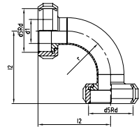
CODO 90° T/T SMS BEND 90° N/N SMS COUDE 90° E/E SMS
